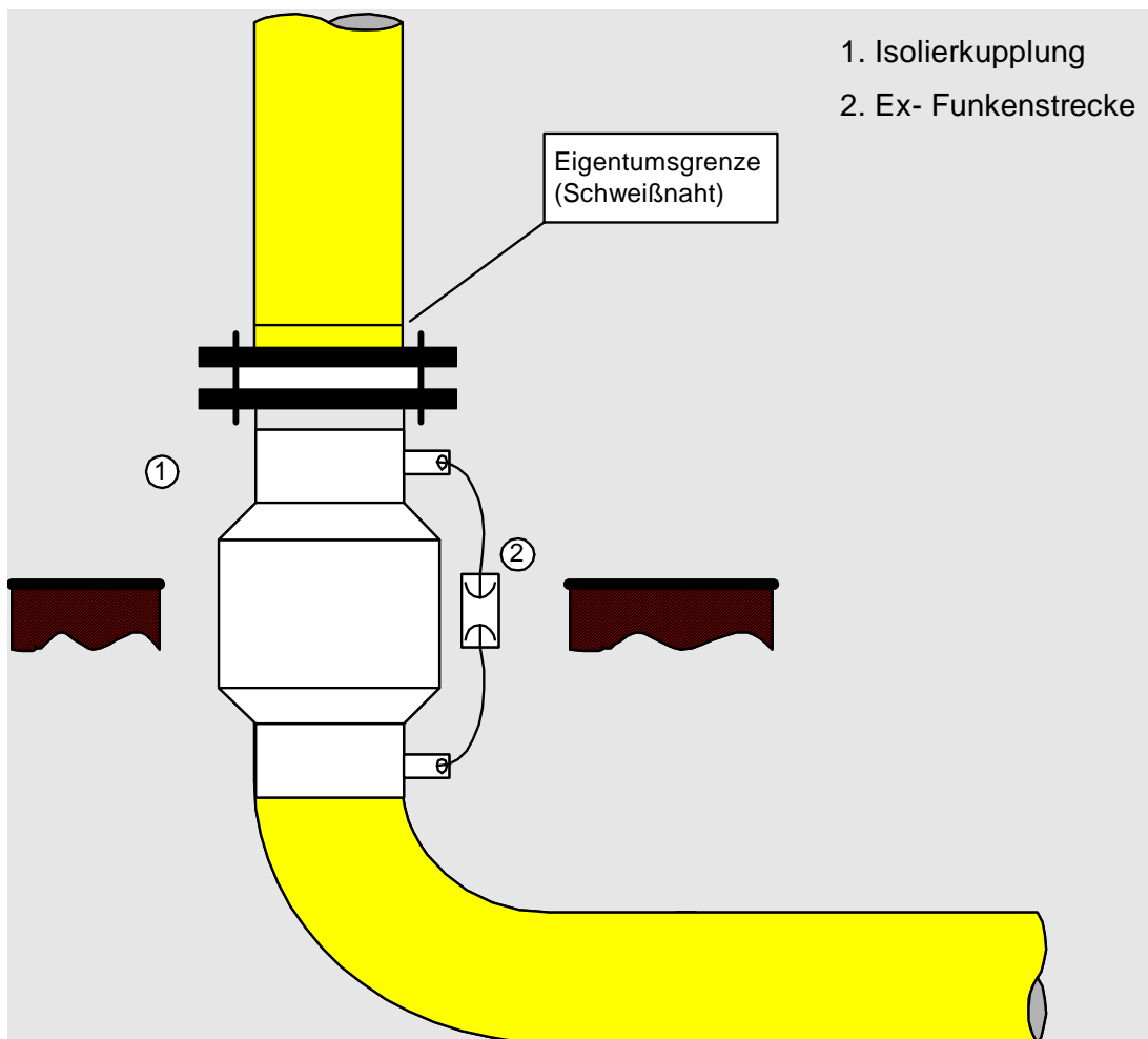
Abbildung 1: Anordnung Einbau Isolierkupplung
